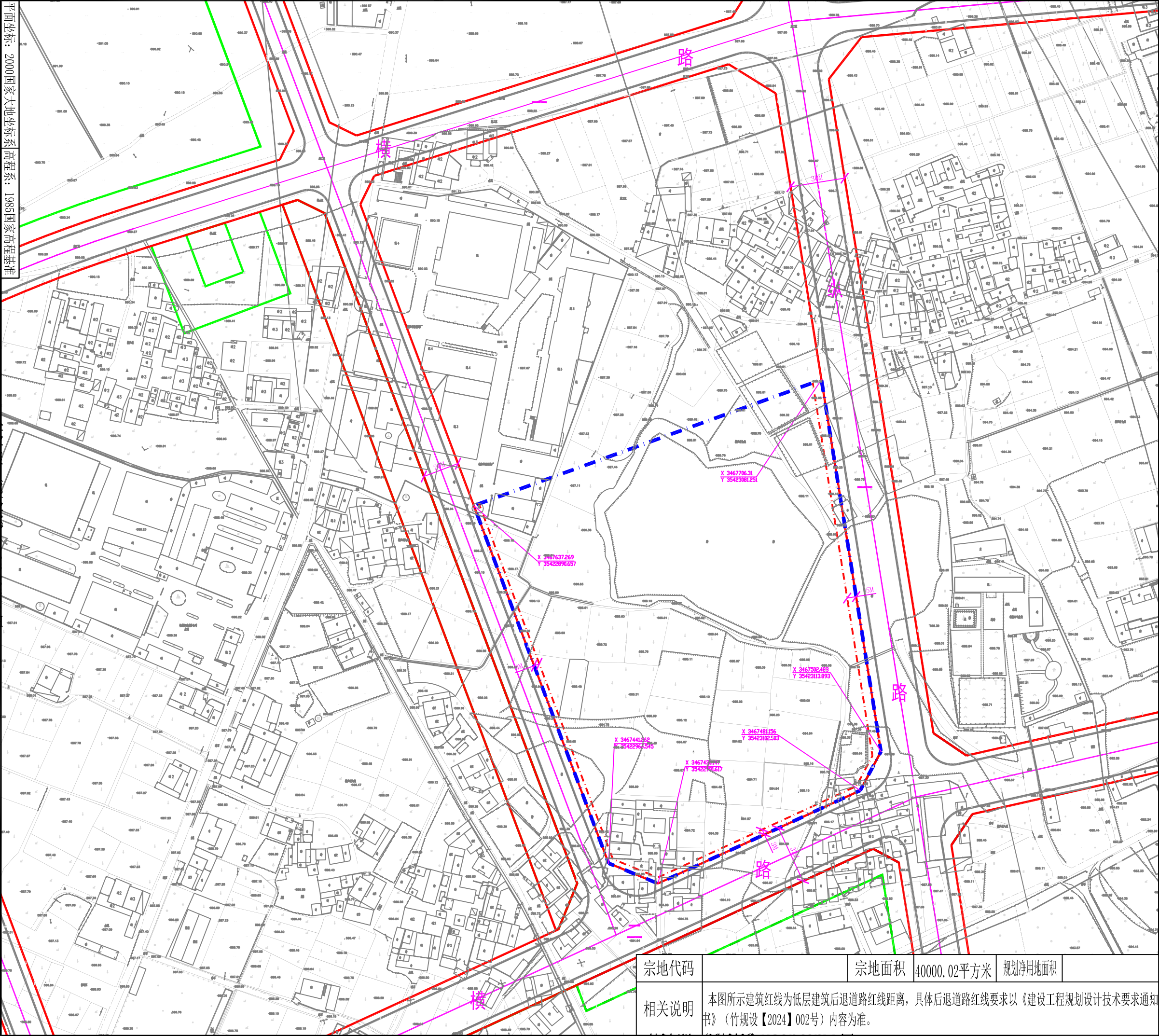
名酒食品工业园MJ-04-07地块内40000.02平方米土地地形红线图
