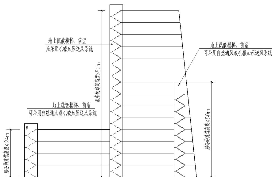
附图 12.2.1 防烟系统设置示意图
