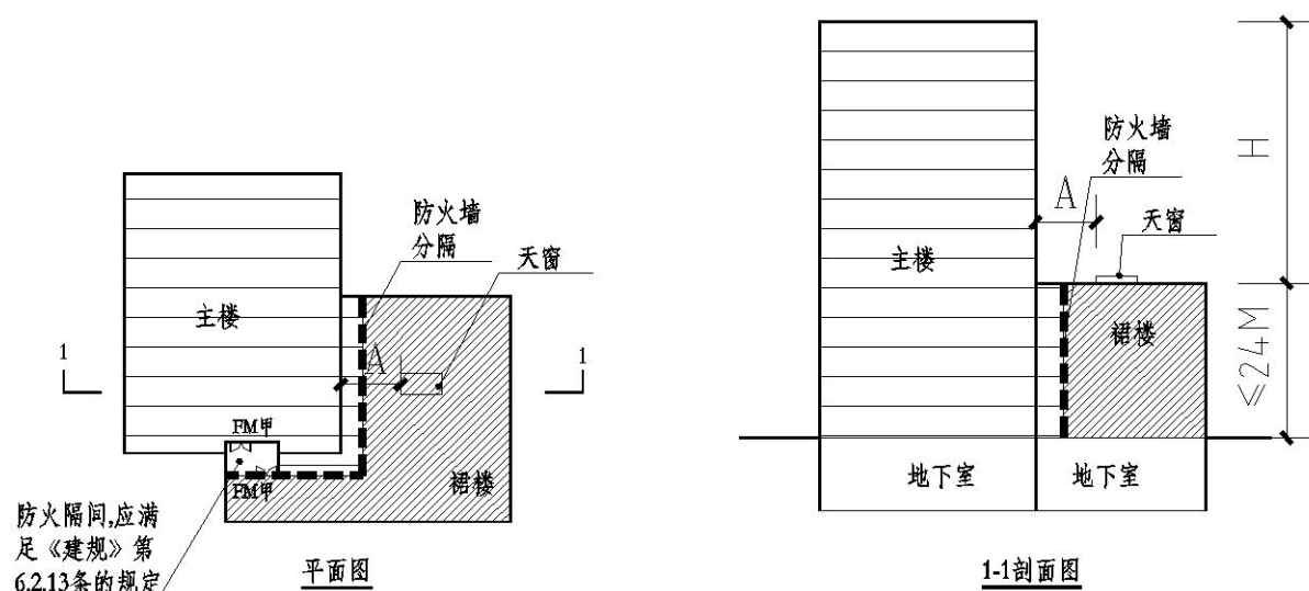
附图 4.1.1-2 高层与裙房分隔示意图（二）
