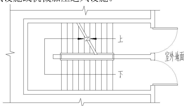
附图 12.2.3 不共用楼梯首层平面示意图
