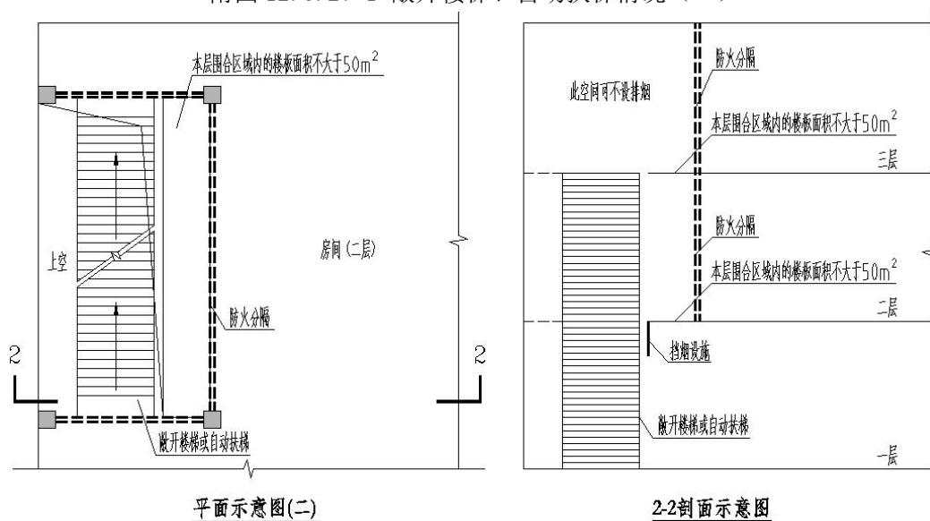
附图 12.3.27-2 敞开楼梯、自动扶梯情况（二）
