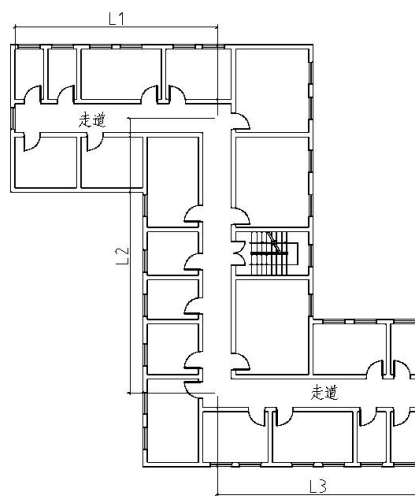
防烟分区长边 L_{\text{长边}} = L1 + L2 + L3 附图 12.3.8-2 “Z”形走道
