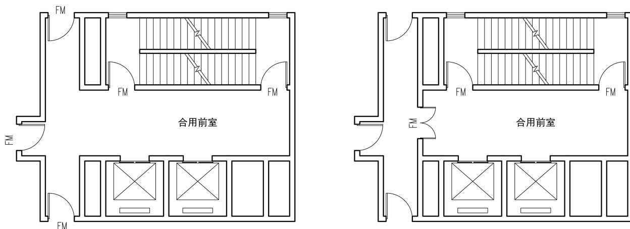
附图 6.2.2-2 同层户门在 3 幢及以下时
