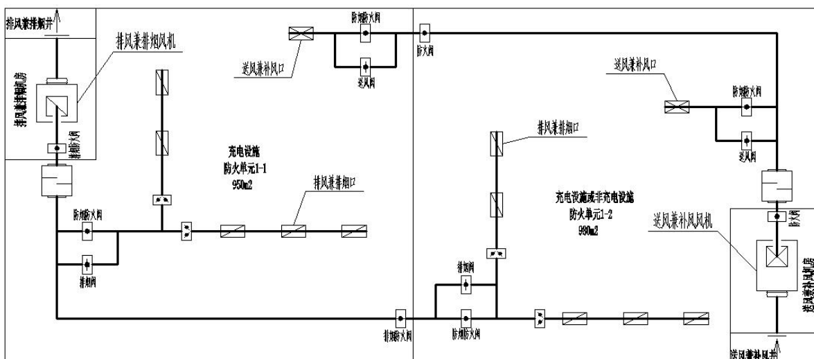
附图 12. 3. 28 汽车库防火单元的通风及排烟平面示意图
