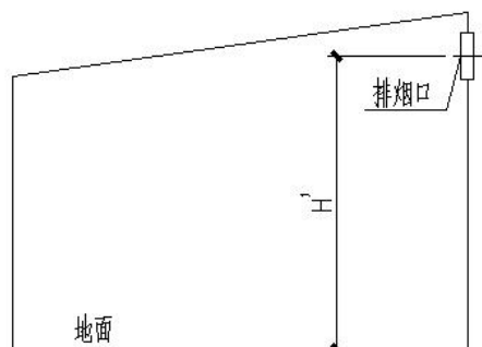
附图 12.3.11-4 斜坡屋顶（坡顶侧墙面排烟）
