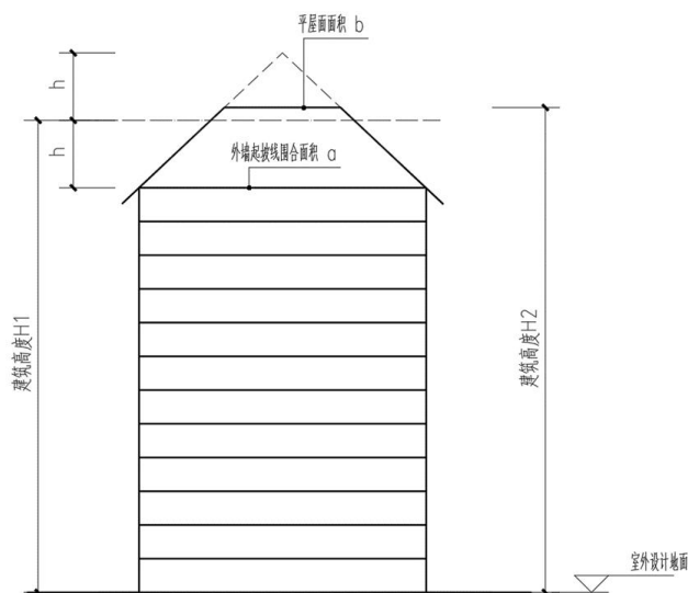
附图 4.2.1-3 平-坡结合屋顶建筑高度计算
