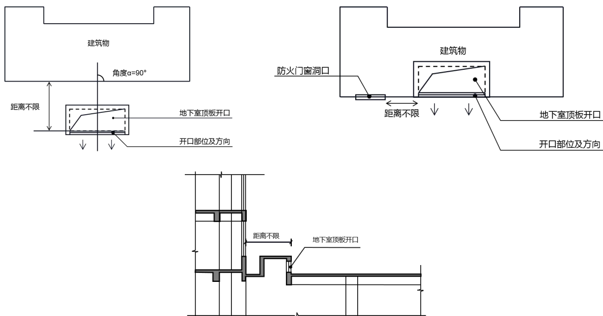
附图 5.3.2-2 地下室顶板开口背向建筑物
