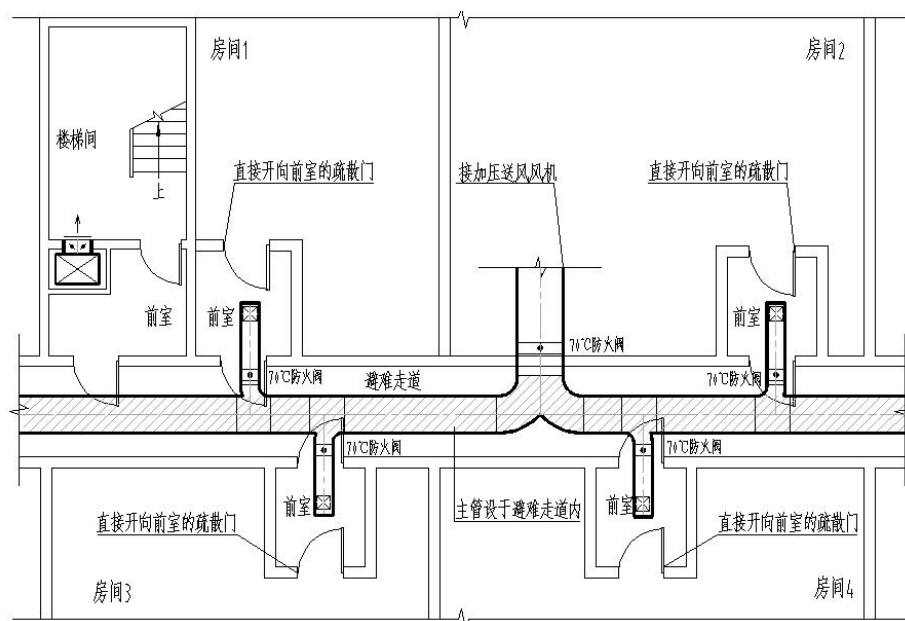
附图 12.2.7 同一避难走道的多个前室合用加压送风系统的送风主管设置
