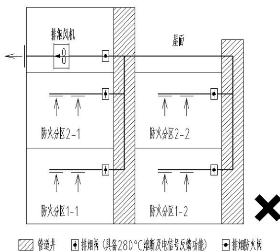
附图 12.3.20 竖向排烟系统错误做法示意图
