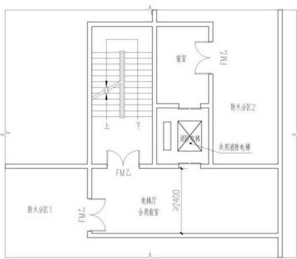
附图 8.4.3-2 消防电梯共用
