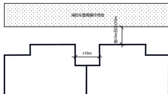
附图 5.2.4-2 建筑凹进部分的宽度不大于 10m 时
