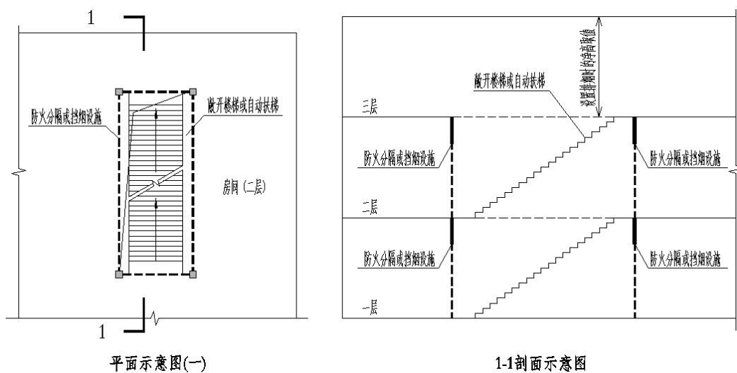
附图 12.3.27-1 敞开楼梯、自动扶梯情况（一）
