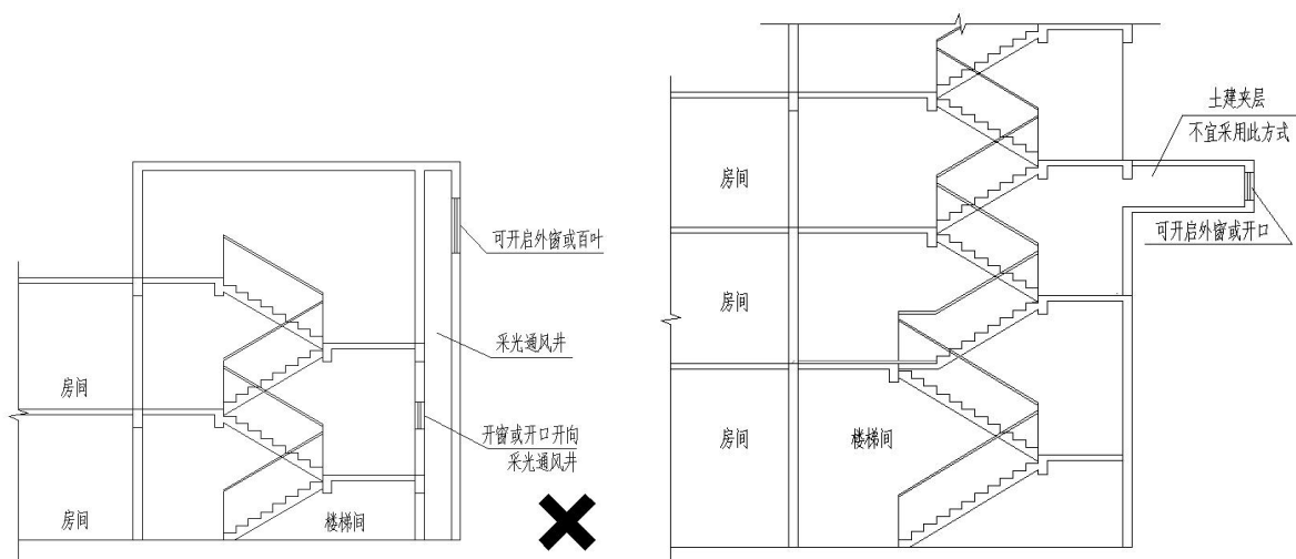
附图 12.2.4-3 不得采用采光通风井方式
