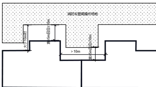
附图 5.2.4-1 建筑凹进部分的宽度大于 10m 时
