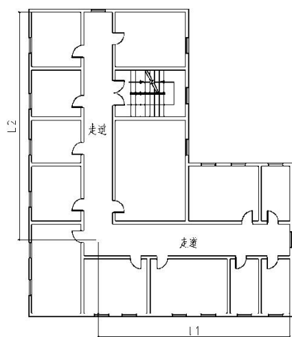
防烟分区长边 L_{\text{长边}} = L1 + L2 附图 12.3.8-1 “L”形走道
