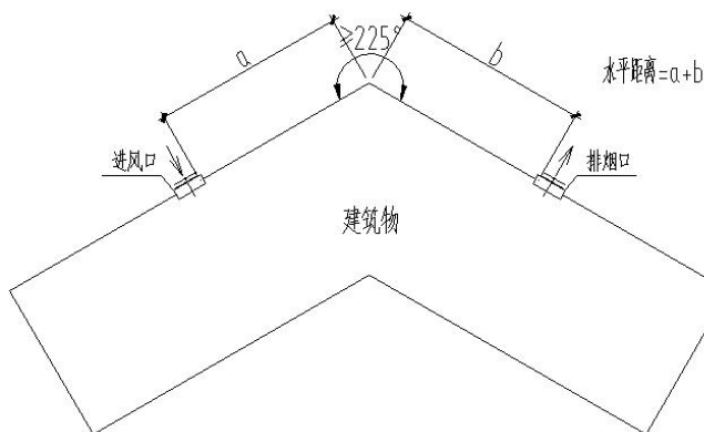
附图 12.2.14-2 进、出风口布置平面示意图
