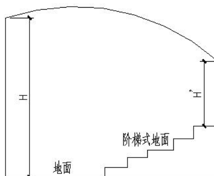
附图 12.3.11-6 阶梯式地面场所
