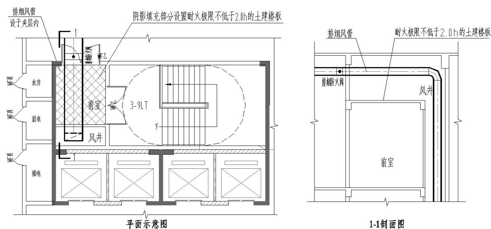
附图 12.4.5 排烟管道水平通过前室的做法示意
