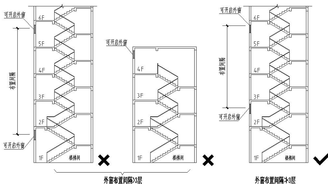
附图 12.2.4-5 自然通风外窗布置间隔示意
