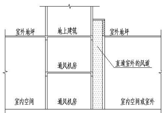
附图 12.4.2-1 直通室外的风道示意
