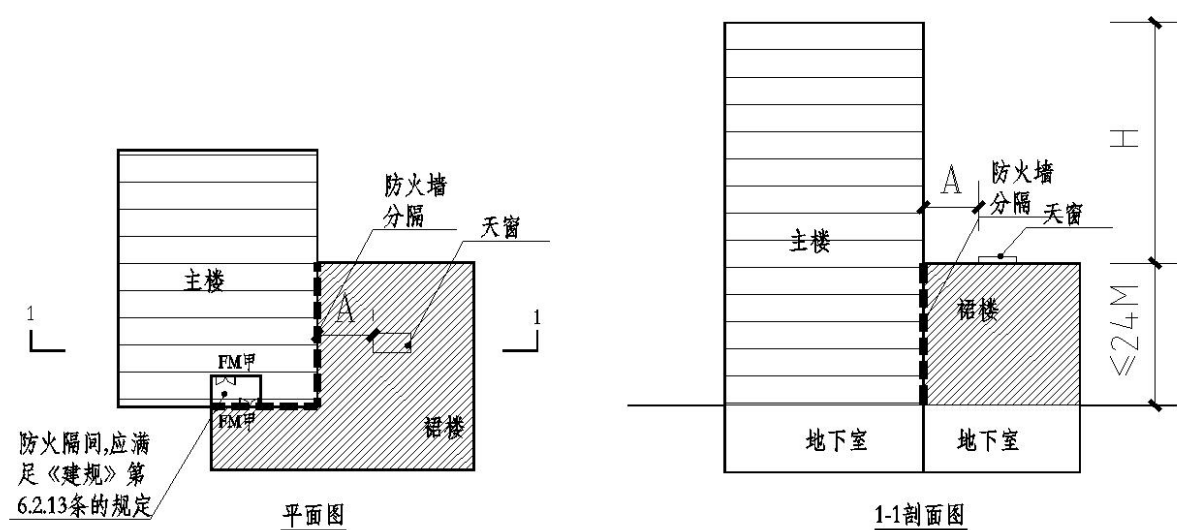
附图 4.1.1-1 高层与裙房分隔示意图（一）
