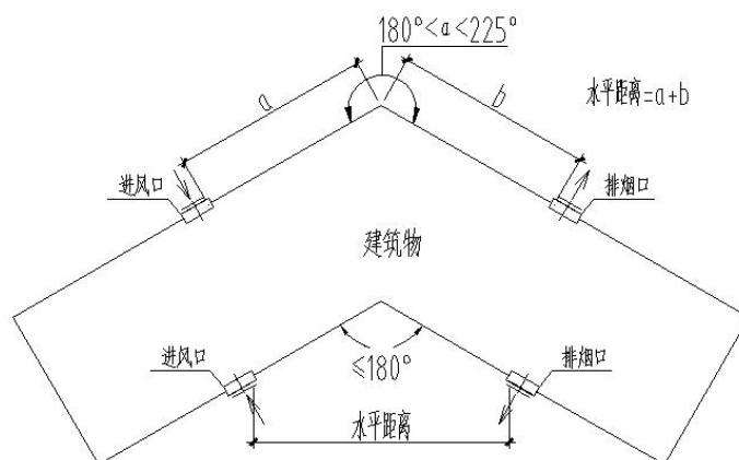
附图 12.2.14-1 进、出风口布置平面示意图
