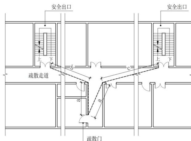
附图 7.2.1 丁字型走道疏散距离
