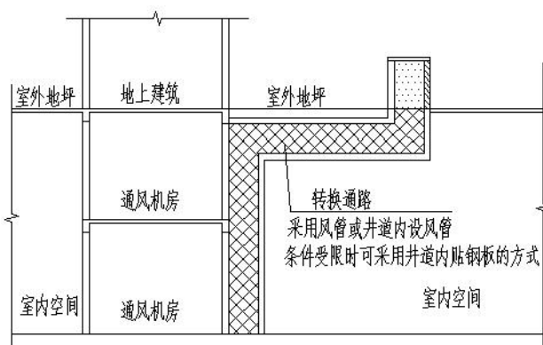
附图 12.4.2-2 转换通路示意
