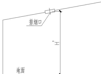
附图 12.3.11-2 斜坡屋顶（顶排烟）
